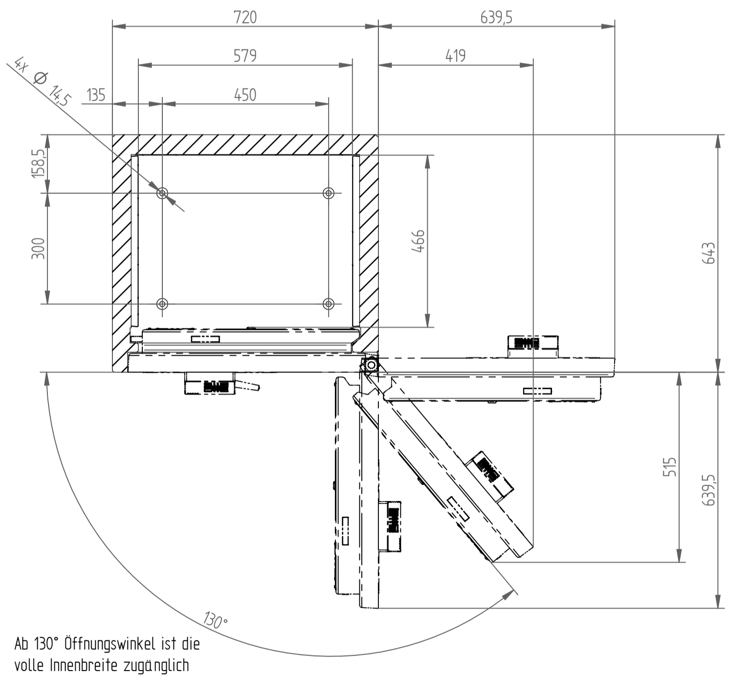
Schnitt A-A
